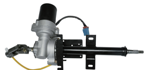
Steering Column 转向管柱
