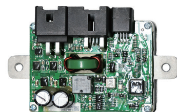
Electronic Control Unit(ECU) 控制器
